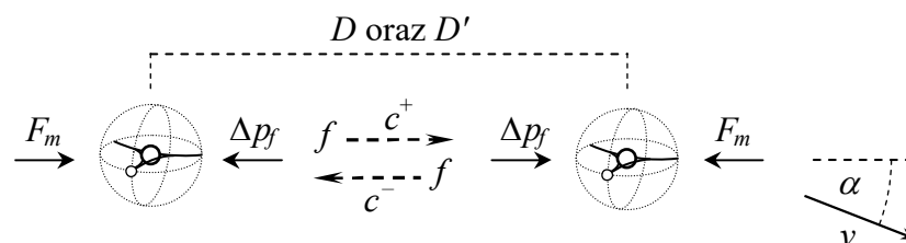
Rys. 1. Na atomy działają dwa przeciwstawne oddziaływania.
