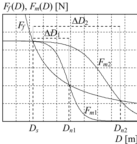
Rys. 5. Przykład ciała kruchego ( F_{m1} ) oraz ciągliwego ( F_{m2} ).
