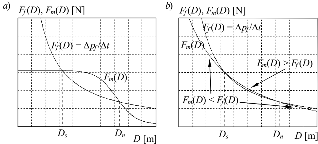
Rys. 2. Przykładowe wartości oddziaływań pomiędzy atomami ciała stałego dla ustalonej wartości prędkości v .
