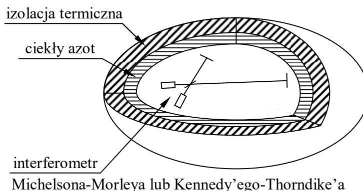
Rys. 7. Propozycja eksperymentu, którego celem jest zmierzenie naszej prędkości względem eteru [76]. Jeżeli interferometr jest schłodzony do niskich temperatur, wtedy w jego ramionach nie ma ciśnienia fotonowego, które zależy od prędkości względem eteru. Schłodzone ramiona nie będą podlegały skróceniu Lorentza-Fitzgeralda, dlatego schłodzony interferometr może pokazać wynik pozytywny pomiaru naszej prędkości względem eteru.
