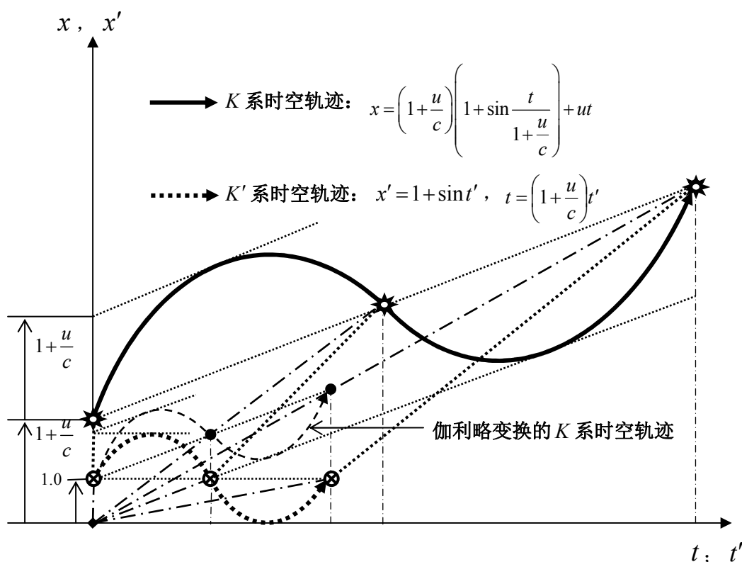
图 10 在 x 轴方向上 K' 系时空轨迹与 K 系时空轨迹之间的 ‘协变’
