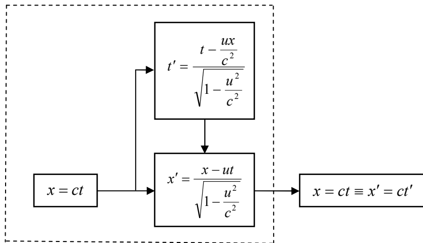
图 3 时空轨迹 x = ct 在“洛伦兹变换”下的“协变”
