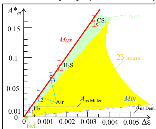
Рис.1. Зависимость A_m(\Delta \epsilon) амплитуды A_m сдвига интерференционной полосы от поляризационного вклада \Delta \epsilon частиц в полную проницаемость \epsilon = 1 + \Delta \epsilon светоносной среды интерферометра Майкельсона (ИМ), обнаруженная мной в 1968 году [2]:
