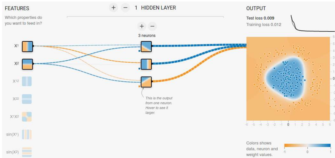
图 3. 神经网络，一种特殊的集成分类器
