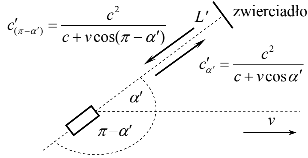
Rys. 5. Prędkości światła w eksperymentach Michelson'a-Morley'a.
