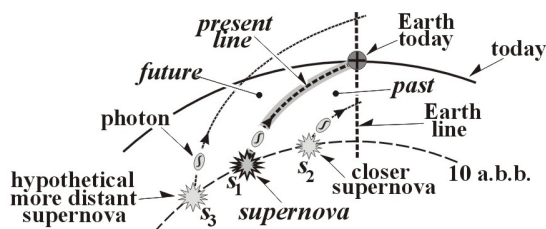
Fig. 0-16. Supernovas.
