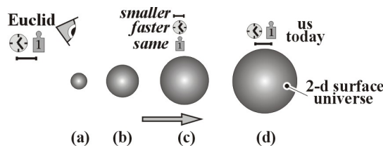
Fig. 0-23. Big Bang (2)
