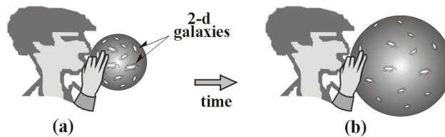
Fig. 0-17. 2-d universe (2).
