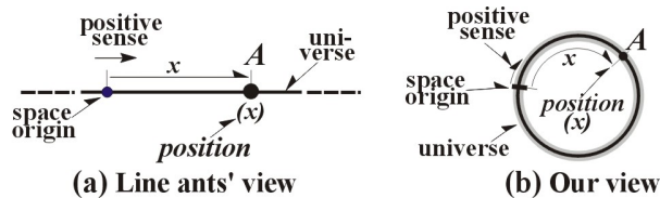
Fig. 0-3. Position.
