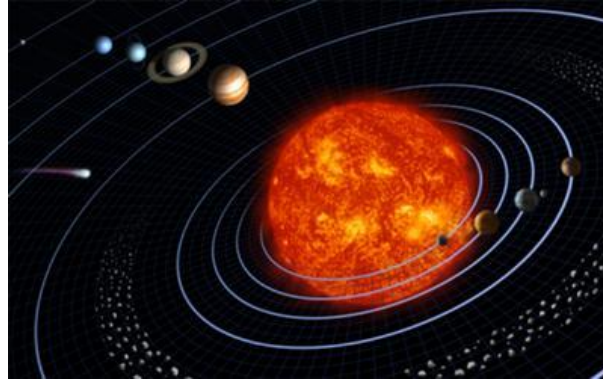
Рис.1. Солнечная система, вид сверху.
