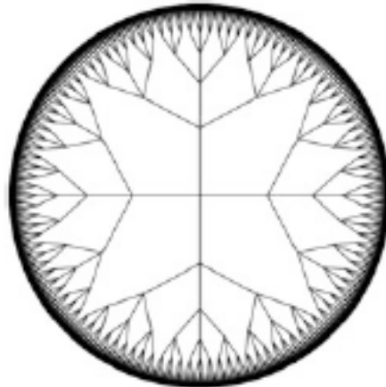
P^1(Q_3)
