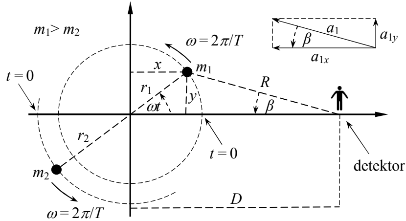
Rys. 1. Dwa ciała o masach m_1 oraz m_2 wirujące po okręgach o promieniach r_1 oraz r_2 .
