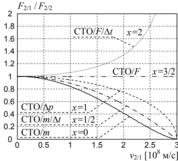
Рис. 6. Зависимости между измерениями одинаковой силы двумя различными наблюдателями в динамиках моделей:
