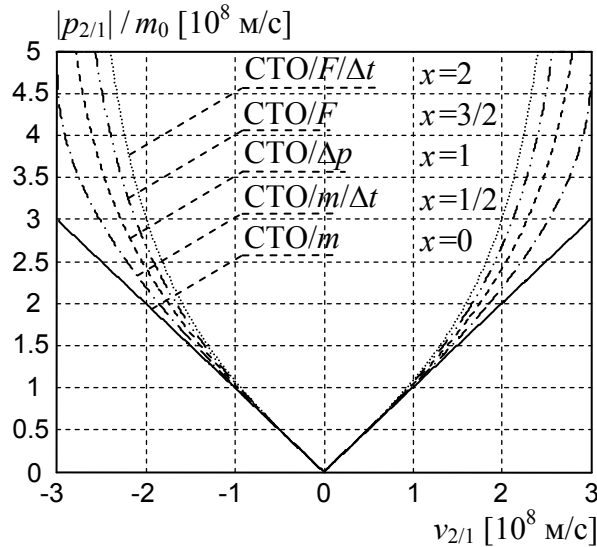
Рис. 4. Модуль импульса в динамиках моделей: СТО/ m ( x=0 ), СТО/ m/\Delta t ( x=1/2 ), СТО/ \Delta p ( x=1 ), СТО/ F ( x=3/2 ) и СТО/ F/\Delta t ( x=2 ).
