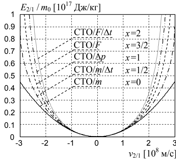
Рис. 5. Кинетическая энергия в динамиках моделей: STO/m ( x=0 ), STO/m/Δt ( x=1/2 ), STO/Δp ( x=1 ), STO/F ( x=3/2 ) и STO/F/Δt ( x=2 ).
