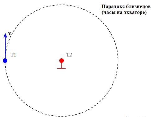
Рис.4 С точки зрения движущихся часов T2 вокруг них по окружности движутся неподвижные часы T1.
