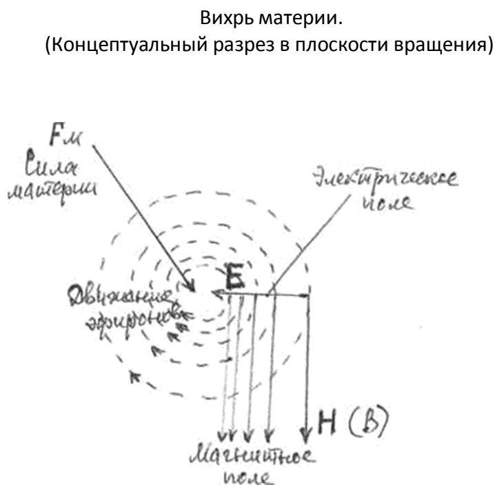
Рис. 3. Принцип возникновения силы материи и её электромагнитная суть, а, заодно, и суть электрического и магнитного полей.
