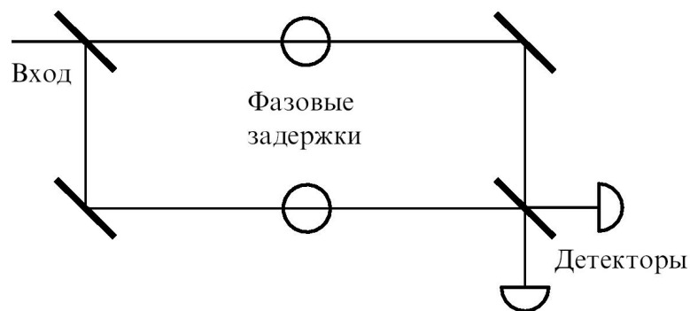
Рис.3. Схема интерферометра Маха-Цандера.
