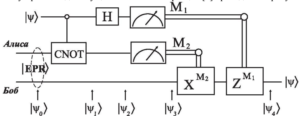
Рис.6. Схема установки для осуществления квантовой телепортации состояния фотона
