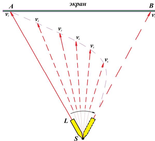
Рис.1. Источник L излучает единичные фотоны \nu в сторону экрана АВ. По экрану перемещается не «световой зайчик», а несвязанные фотоны создают каждый раз нового «светового зайчика»
