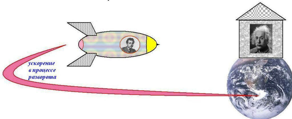
Рис.1. Парадокс близнецов
