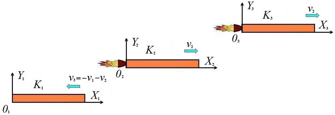
Рис.4 Три системы отсчета, движущиеся друг относительно друга.
