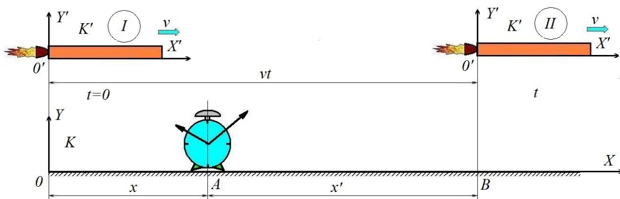
Рис.2 В неподвижной инерциальной системе отсчета K часы имеют координату x , а в подвижной инерциальной системе отсчета K' по истечении времени t - координату x' .
