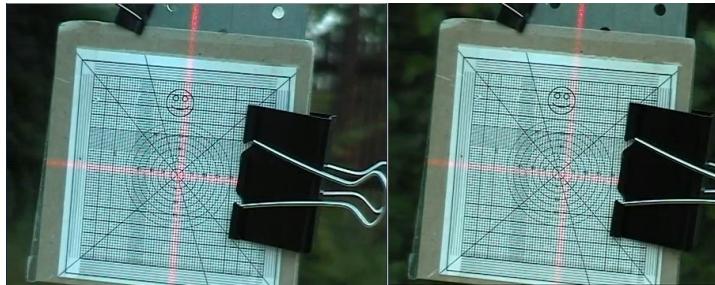
Рис.6 Кадры из видеоклипа В.Приставко в эксперименте с поворотом платформы вокруг вертикальной оси. Кадры отобраны «на глазок», по их номерам. Считаем, что они соответствуют двум положениям балки, отстоящим друг от друга на 90 градусов.
