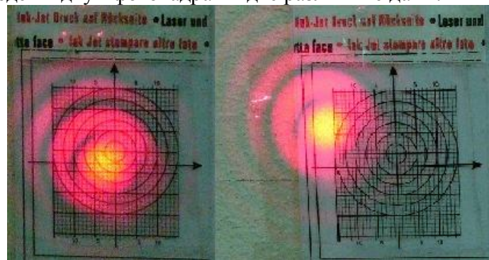
Рис.8 Фотоснимки В.Приставко в эксперименте с неподвижным лазером и мишенью, расположенными на расстоянии ок.32 м друг от друга. Кадры получены 7 мая и 20 мая.
