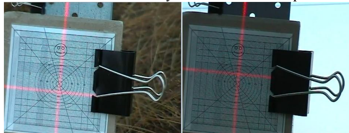
Рис.7 Кадры из видеоклипа В.Приставко в эксперименте с поворотом платформы вокруг горизонтальной оси. Кадры отобраны «на глазок», по их крайним положениям (максимальным отклонениям) вверху и внизу.
