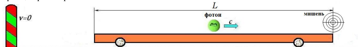
Рис.10 Схема условно неподвижной ИСО. Длина платформы - L . Фотон преодолевает это расстояние (от начала платформы до мишени) за время t .
