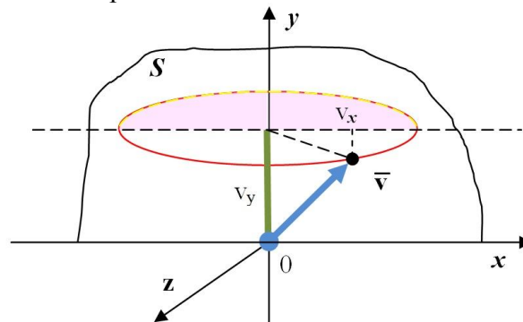
Рис.14. Схема, показывающая, как вращается вектор скорости в системе отсчета платформы в эксперименте В.Приставко с поворотом платформы вокруг вертикальной оси. Проекция вектора скорости на ось вращения имеет неизменное значение.
