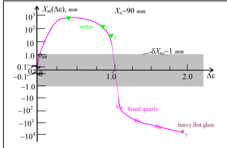
Рис.4. Зависимость амплитуды X_m гармонического сдвига интерференционной полосы от вклада \Delta\varepsilon диэлектрической проницаемости частиц светоноса в полную диэлектрическую проницаемость \varepsilon=1+\Delta\varepsilon оптической среды: воздуха, воды, плавленого кварца и стекла «тяжелый флинт» из [13 1 ]. Измерения проведены на разных интерферометрах: с газовыми светоносами при длине плеч L=L_1=L_2=6 м; для светоносов из воды и твёрдых сред длина плеч была L=0.3 м. Точки 1, 4; 2, 5 и 3, 6, 7 измерены на длинах волн: 9 \cdot 10^{-6} , 9 \cdot 10^{-7} и 3 \cdot 10^{-7} м, соответственно, а измерения на газах велось на длине волны света \lambda=6 \cdot 10^{-7} м. X_0 – ширина полосы; \Delta X_{ns} – уровень шума интерферометра (все экспериментальные данные приведены к одному размеру L=6 м и к длине волны \lambda=6 \cdot 10^{-7} м). В формулах (2), (3), (6): A_m = X_m/X_0 .
