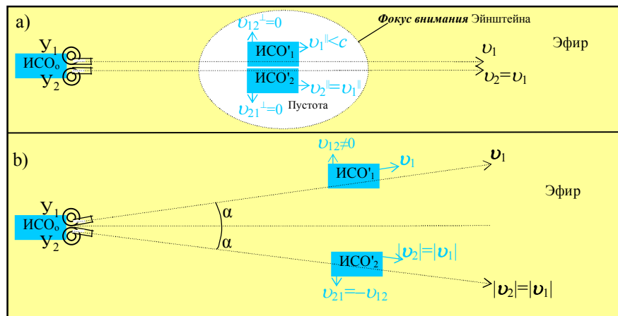
Рис.3. Доказательство экспериментами на ускорителях релятивистских частиц (мюонов и пионов) ошибочности Эйнштейновой кинематической интерпретации:
