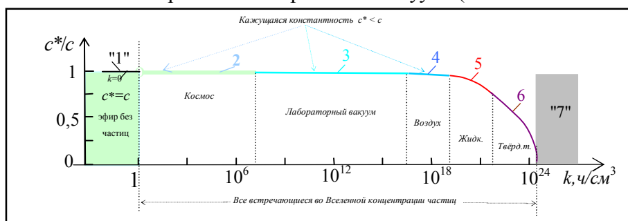
Рис.1. К пониманию кажущейся "независимости" скорости c^*=(\epsilon\mu)^{-1/2} распространения ЭМВ от концентрации ( k, \text{ч/см}^3 ) частиц вакуумных и газовых атмосфер в простейшем линейном масштабе представления оси ординат c^*/c=n^{-1} , где n – показатель преломления среды, в которой распространяется ЭМВ ( n^2=\epsilon\mu/\epsilon_0\mu_0 ).
