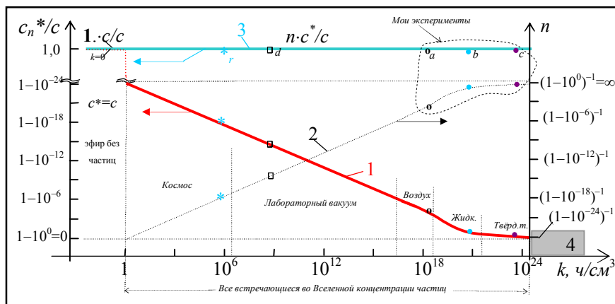
Рис.2. Растянутые двойным логарифмическим масштабом осей абсцисс ( k ) и ординат \{c_n^*(k)/c и n\} зависимости: 1 – относительной скорости c_n^*(k)/c распространения ЭМВ; 2 – показателя преломления n(k) , от концентрации k частиц (поляризующихся атомов) в атмосфере неподвижной ИСО 0 . Константный уровень 3 является произведением соответствующих значений кривых 2 и 1 определяет фактический инвариант \{n \cdot c^*/c\} ЭДТО.
