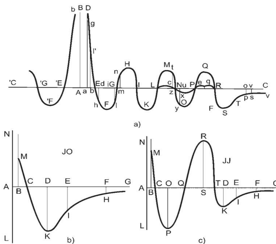
SLIKA 1 – Opšti (a) i posebni oblici (b i c) Boškovićeve krive koja pokazuje promenu privlačne i odbojne sile (donja i gornja ordinata, redom) sa promenom razmaka (apscisa) između elementarnih tačaka ili čestica materije
