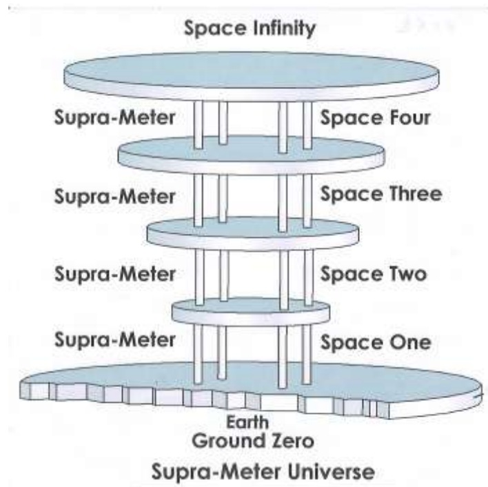
Fig. 3a. The Suprameter Universe
