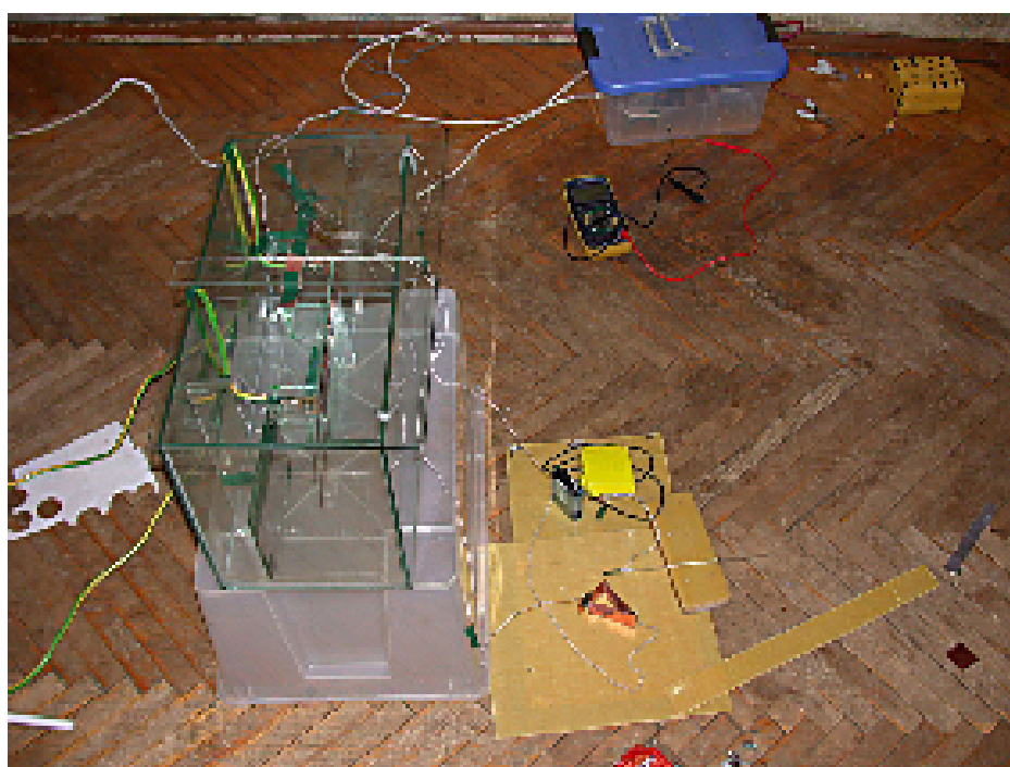
Рис. 11. Экспериментальная установка
