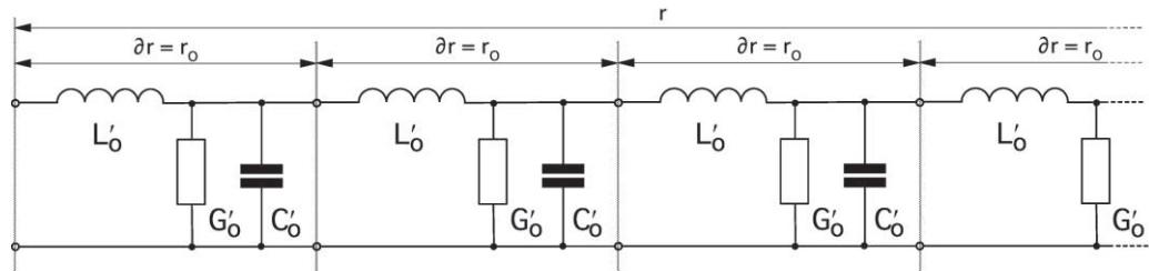
Bild 33 Leitungsersatzschaltung mit Parallelleitwert
