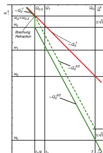
Bild 68a Einkopplungsprozeß
