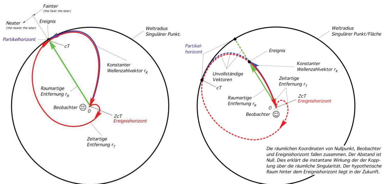
Bild 139 Entfernungsvektoren bei einem Objekt am Rande des Universums (schematisiert)
