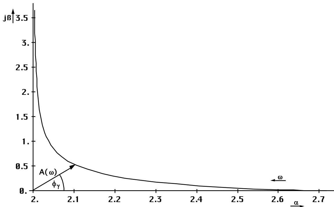
Bild 16 Frequenzgangsortskurve
