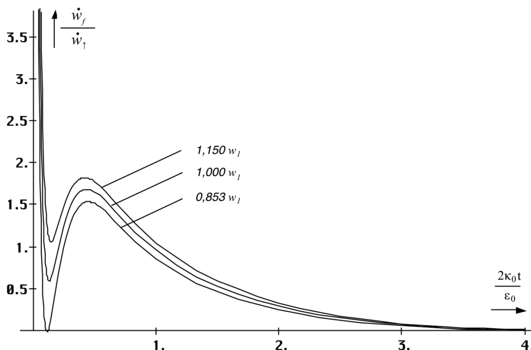
Bild 92 Leistungsdichte Fermionenerzeugung beim Urimpuls
