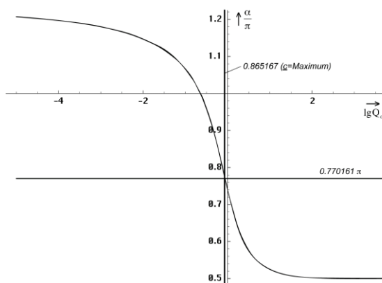
Bild 142 Winkel \alpha als Funktion von Q_0
