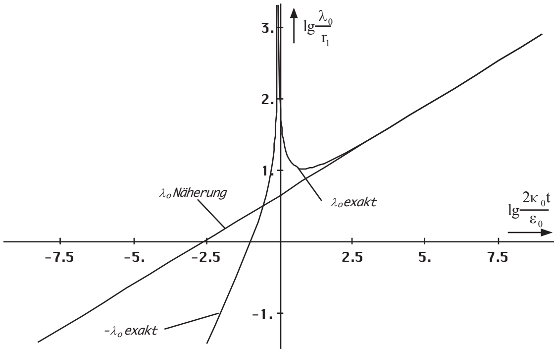
Bild 30 Verlauf von \lambda_0 exakt logarithmischer Maßstab
