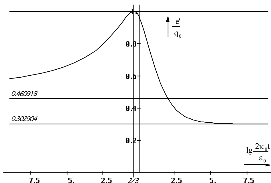
Bild 118 Verhältnis von Elektronenladung und Ladung des MINKOWSKISCHEN Linienelements als Funktion der Zeit/Güte nach (675)
