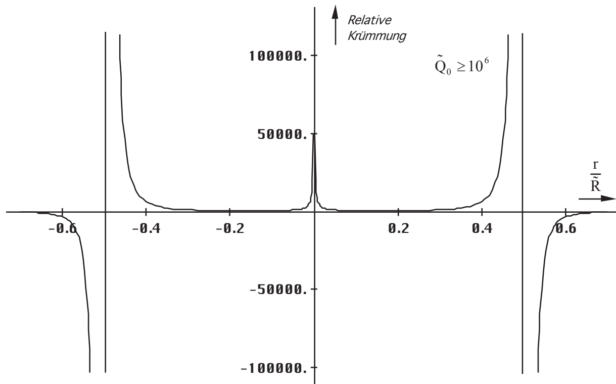
Bild 134 Relative skalare Krümmung für den Standardfall Q_0 > 10^6
