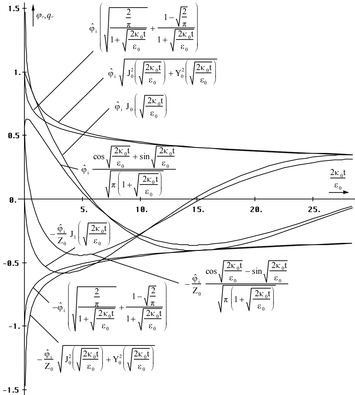
Bild 14 Verlauf von Fluß und Ladung sowie der Nähungs- und Hüllkurvenfunktion (129) in der Nähe der Singularität
