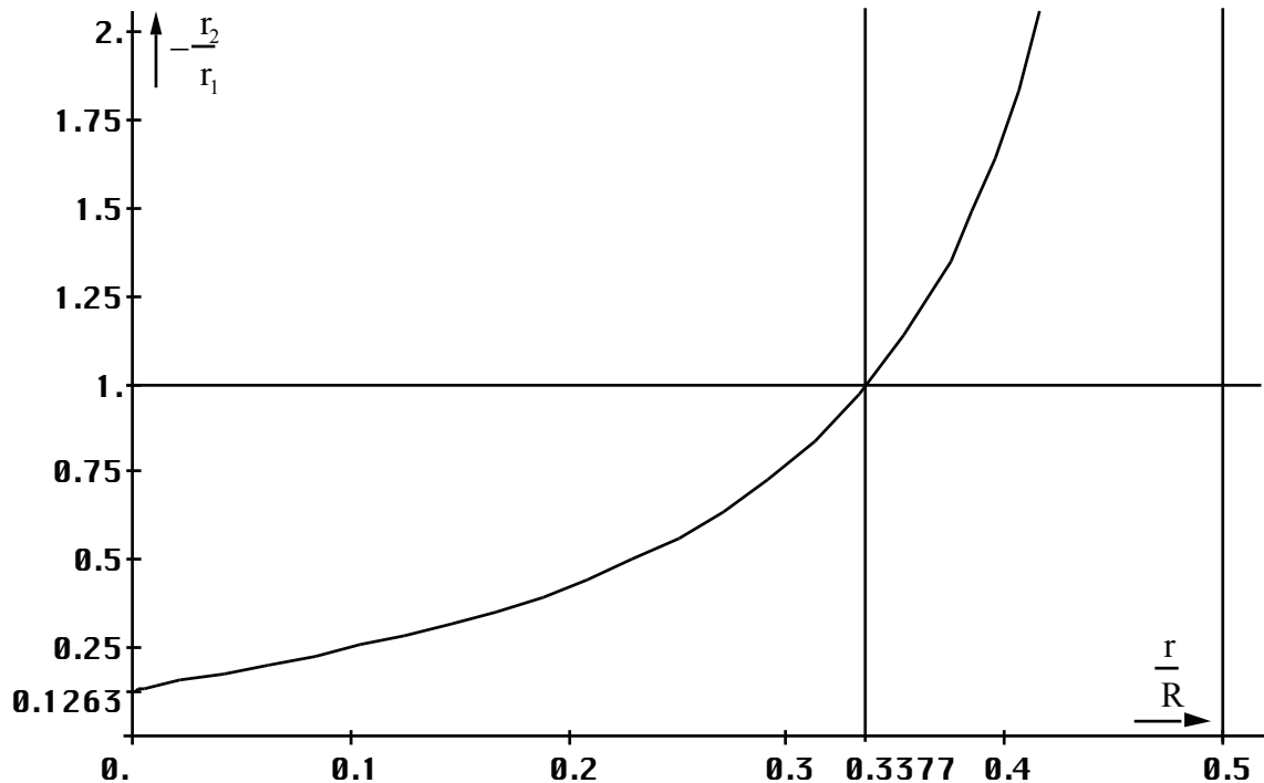
Bild 41 Verhältnis von zweiter und erster Lösung bei t=0
