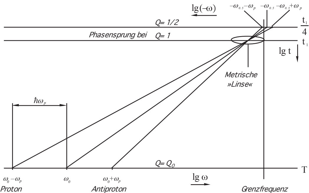
Bild 73 Masse-Rotverschiebung am Beispiel des Protons
