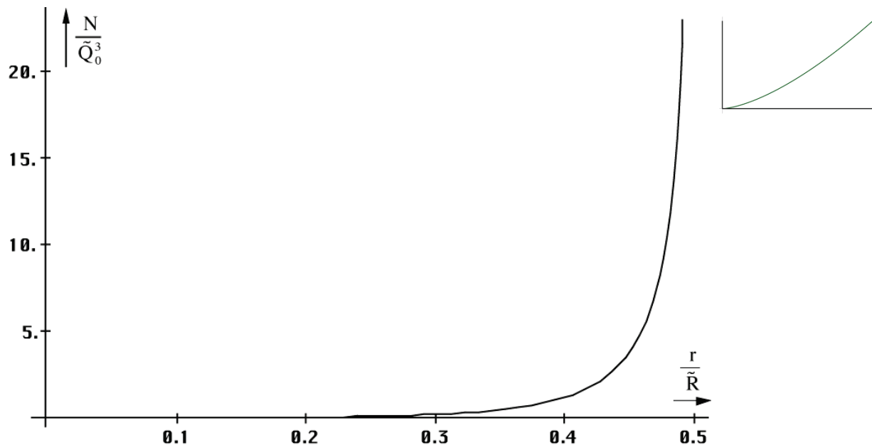
Bild 47 Anzahl MLE's in Abhängigkeit vom Radius
