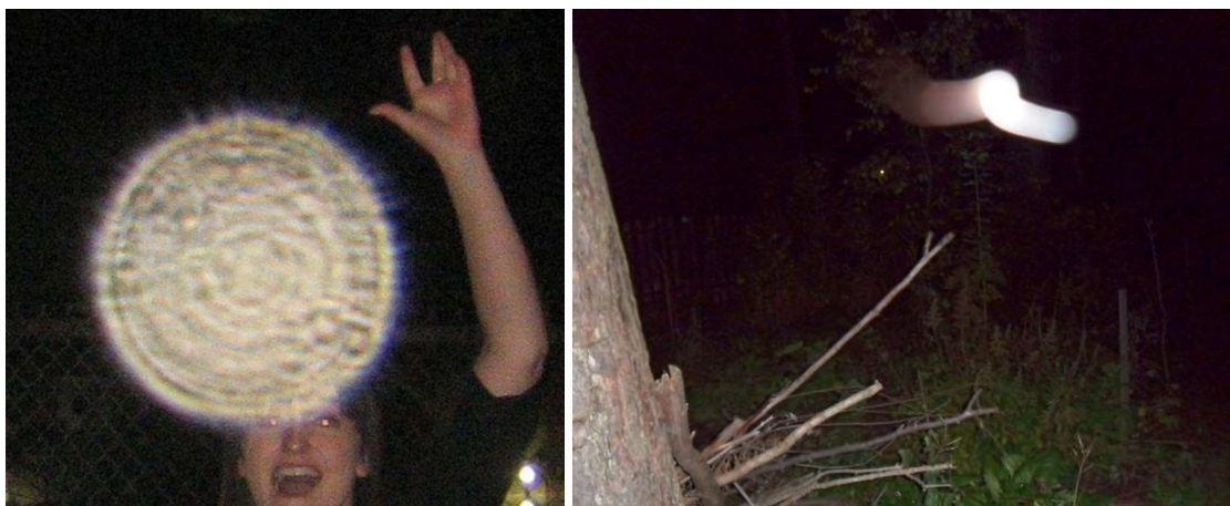
Рис. 7. Тонкое тело в форме сфероида (слева), с его активным перемещением (справа)
