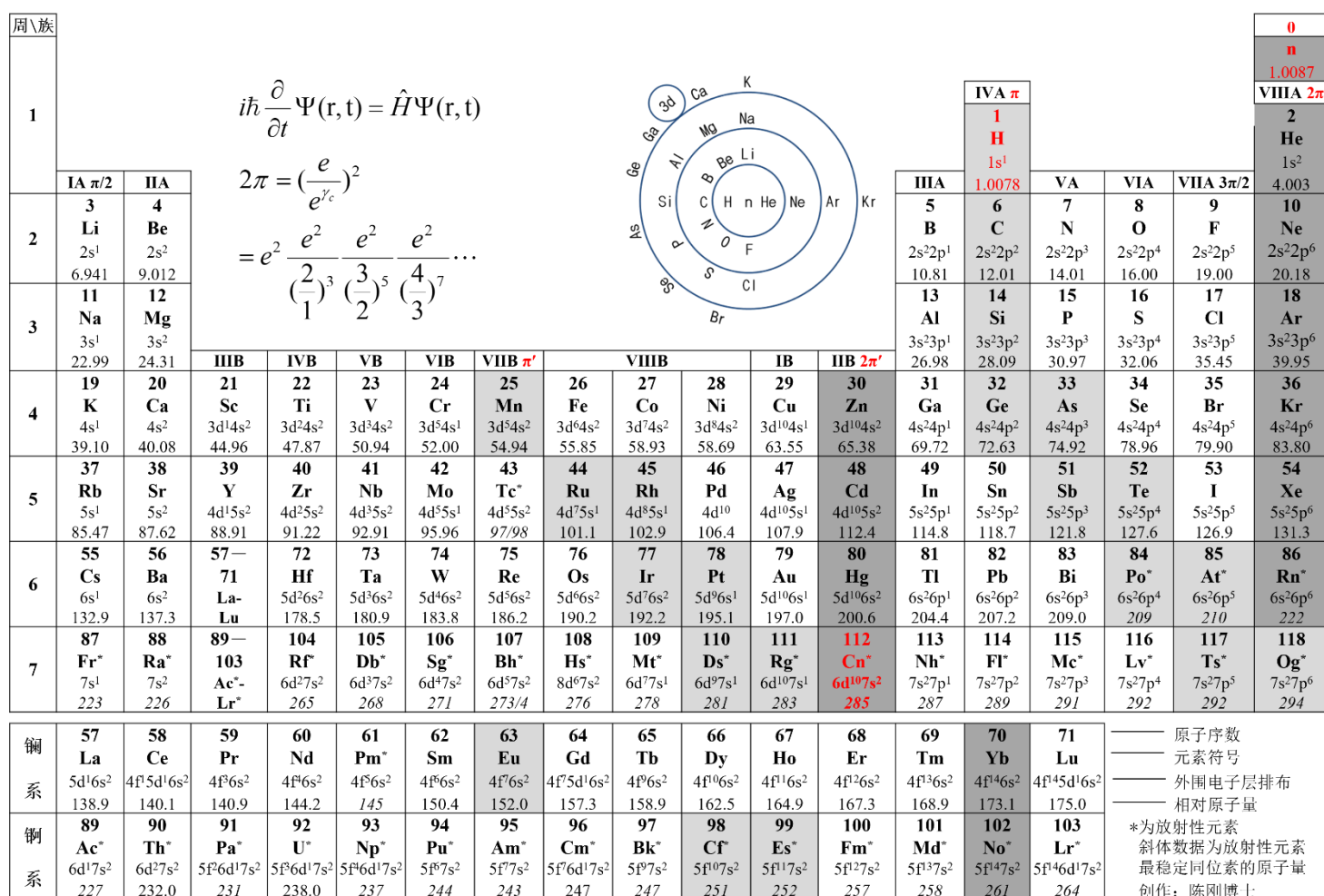
图5. 改进版元素周期表
