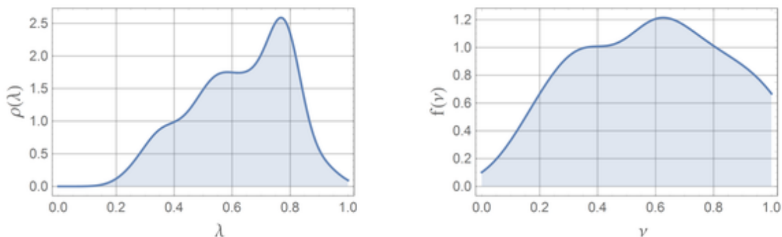
Рис. 3 Функции распределения плотности вероятности \rho(\lambda) и f(v) для Брестской области.
