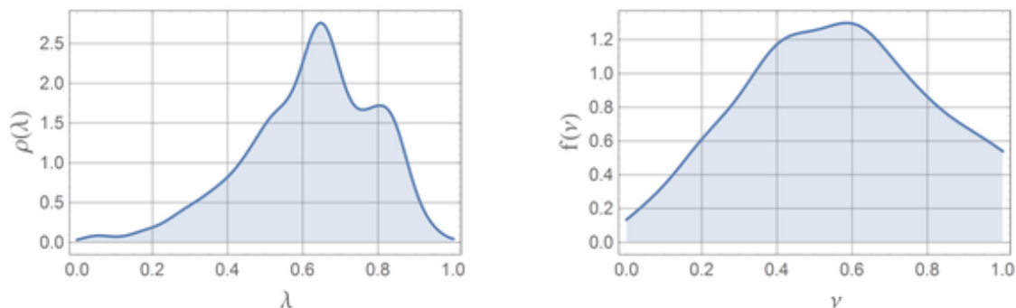
Рис. 1 Функция \rho(\lambda) распределения плотности вероятности процента голосовавших за г-на Лукашенко. Функция f(v) распределения плотности вероятности числа голосовавших за г-на Лукашенко нормированного на среднее число голосовавших на участке, см. (4). Подразумевается некоторый случайный избирательный участок.
