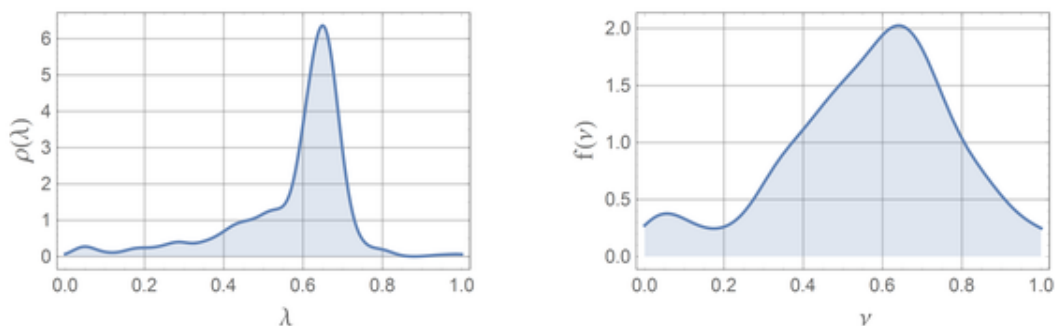
Рис. 2 Функции распределения плотности вероятности \rho(\lambda) и f(v) для Минска.
