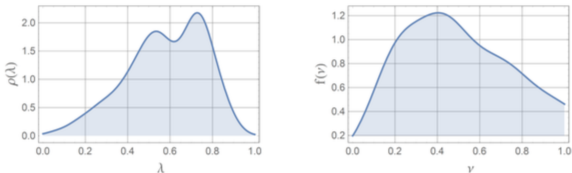
Рис. 7 Функции распределения плотности вероятности \rho(\lambda) и f(v) для Минской области.
