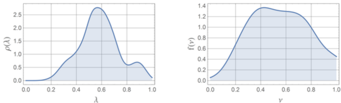
Рис. 6 Функции распределения плотности вероятности \rho(\lambda) и f(v) для Гродненской области.
