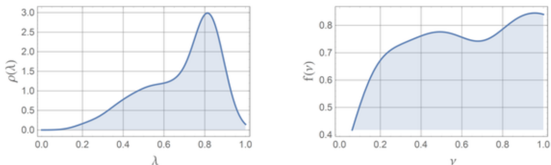
Рис. 5 Функции распределения плотности вероятности \rho(\lambda) и f(v) для Гомельской области.
