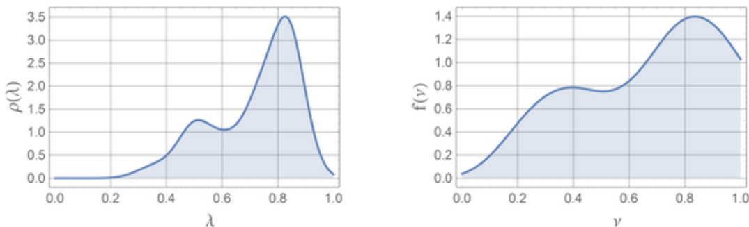
Рис. 4 Функции распределения плотности вероятности \rho(\lambda) и f(v) для Витебской области.
