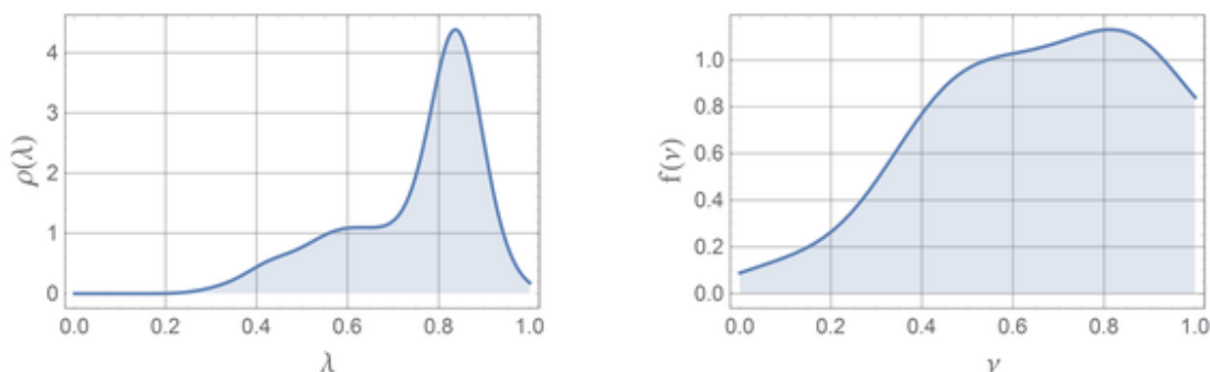
Рис. 8 Функции распределения плотности вероятности \rho(\lambda) и f(v) для Могилевской области.
